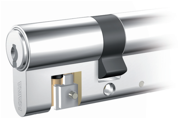
Schnittdarstellung
