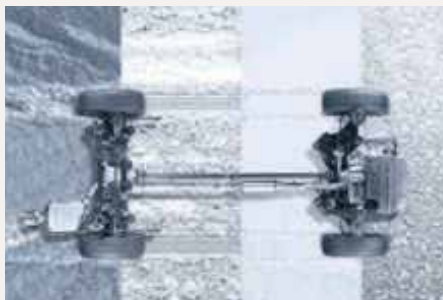
HTRAC-Allradantrieb 1
