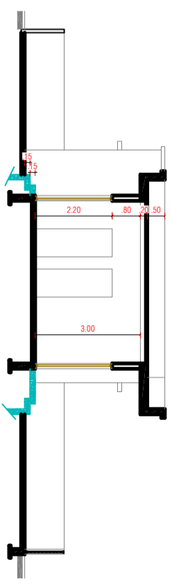
COUPE B-B
