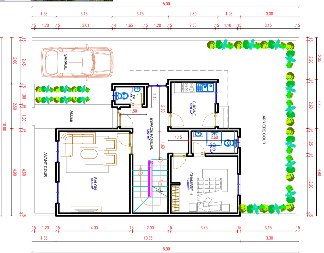
PLAN REZ DE CHAUSSEE
